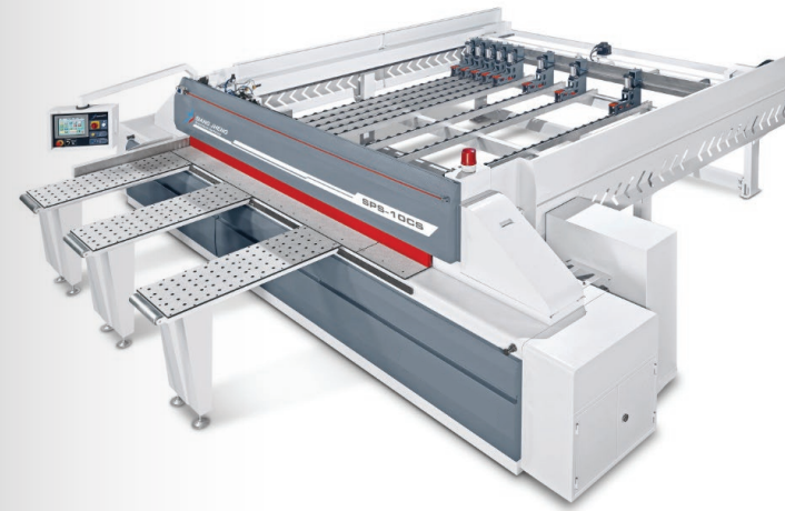
Máy cnc cắt ván công nghiệp tự động
